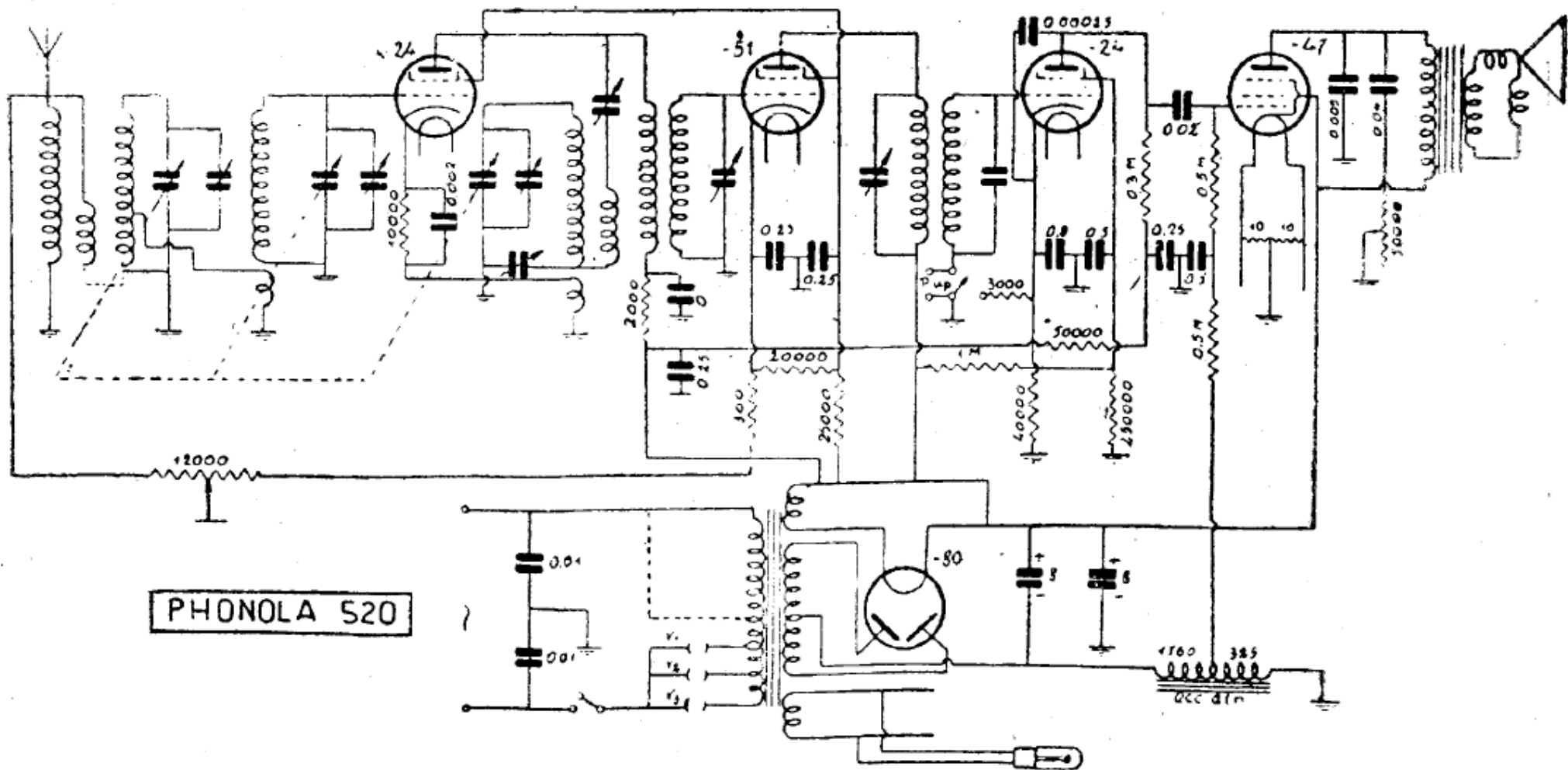
PHONOLA RADIO. — Mod. 520. - Supereterodina con preselettore. - Circuito oscillatore accoppiato al catodo della convertitrice. - MF: 175 kHz. - Produzione 1934.
